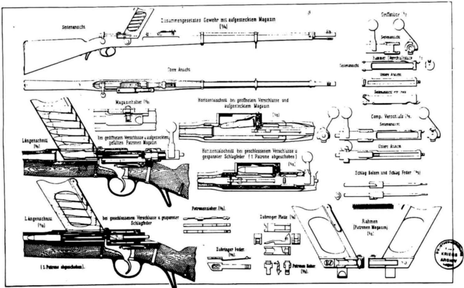
Il Mannlicher modello 1882 con alimentazione dall'alto.
