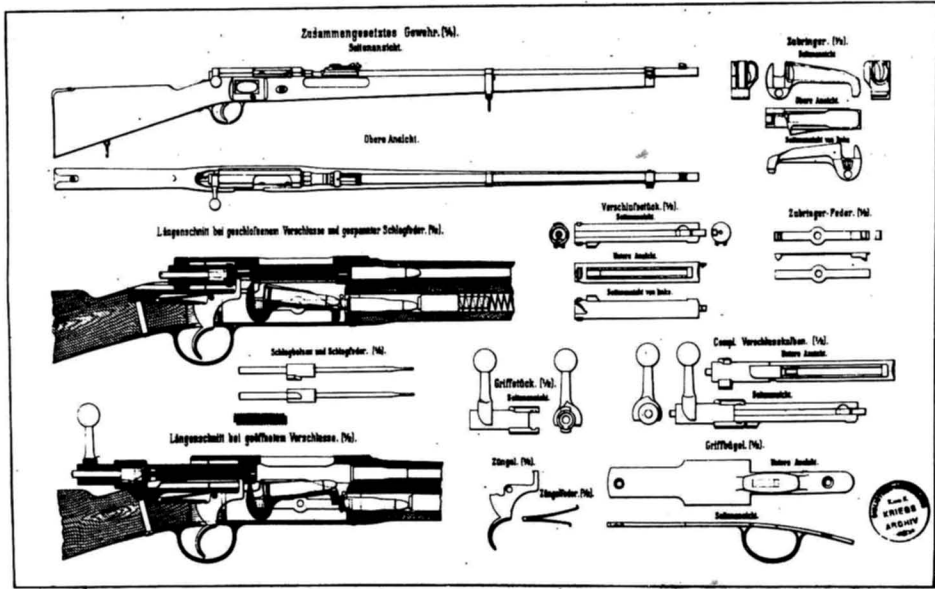
Il Mannlicher modello 1882.
