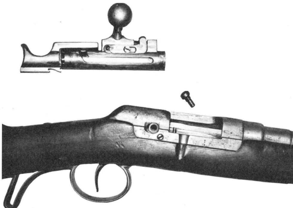
Particolare con l'otturatore estratto.
