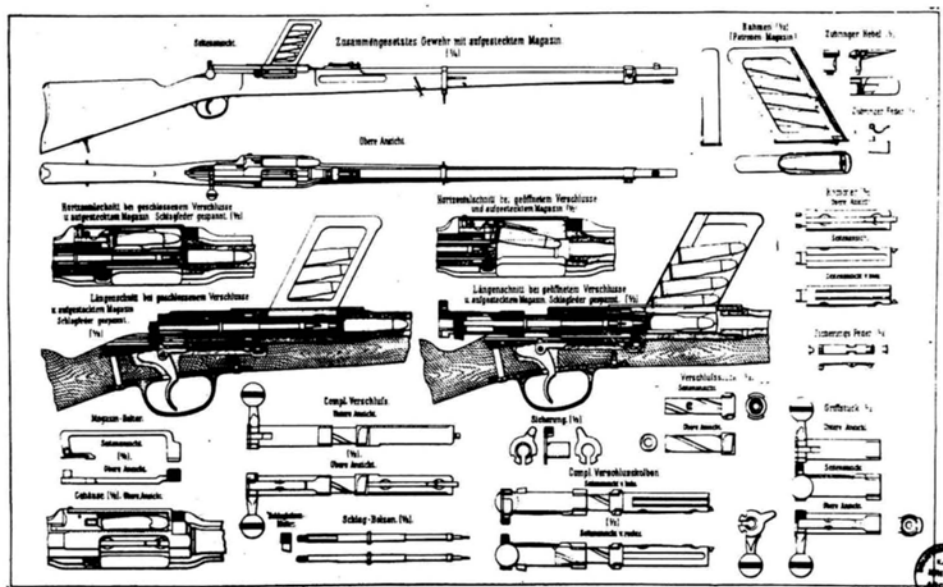
Il Mannlicher modello 1884.
