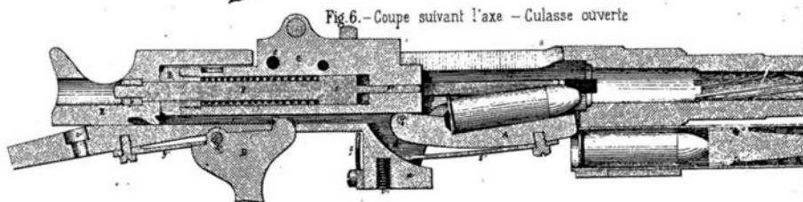
Fig. 6. - Coupe suivant l'axe - Culasse ouverte
