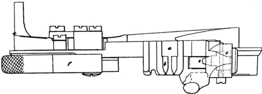
Disegno schematico della batteria Augustin.
