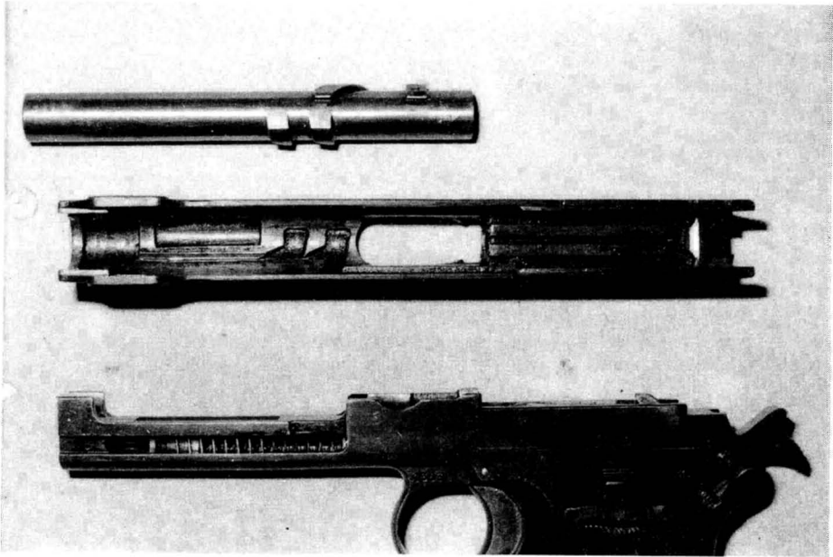
La canna insieme al lato interno del carrello e al fusto. Sotto, il sistema di alimentazione. Notare la molla del cane, la leva di scatto e la molla del disconnettore.
