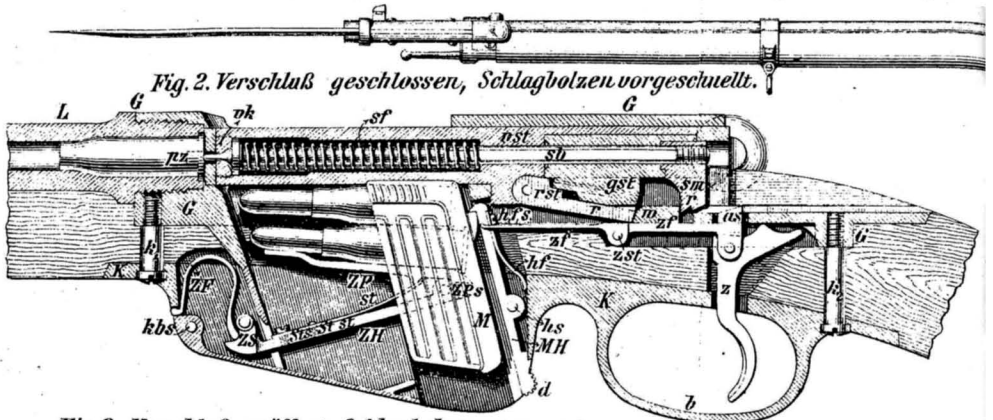
Fig. 2. Verschluß geschlossen, Schlagbolzen vorgeschleift.
