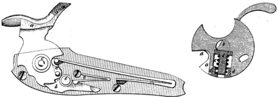
A sinistra, sistema di otturazione M 1873 smontato. In alto, sezione del sistema e disegno della batteria.
