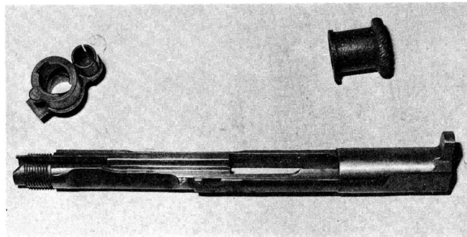
Dall'alto, il castello/culatta con la canna e il percussore, lo stesso con il tappo di volata e il tappo di culatta, e gli stessi elementi rovesciati.
