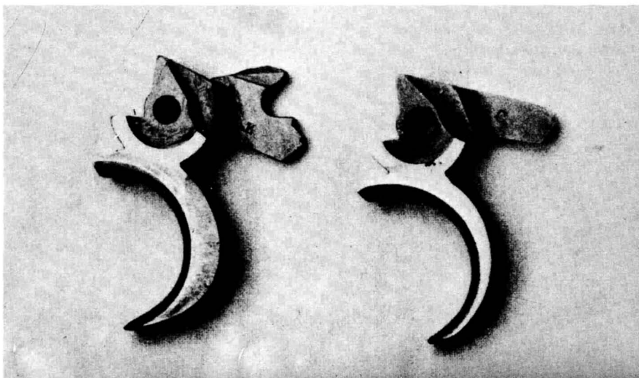
Particolare dello scatto dell'arma priva del disconnettore e i due tipi di grilletto: a destra quello dell'arma priva di disconnettore.
