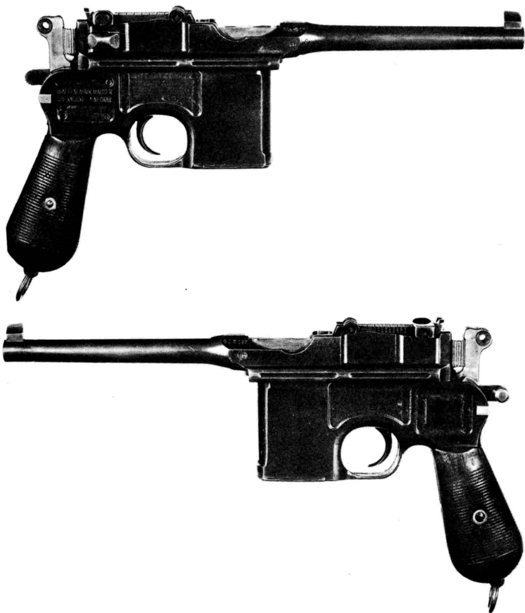
Pistola Mauser M 1896 per la Marina Imperial-Regia, lato destro e lato sinistro. Per una completa descrizione di questo modello vedere l'appendice I.
