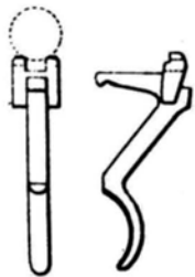
Zügel. (1/2).
