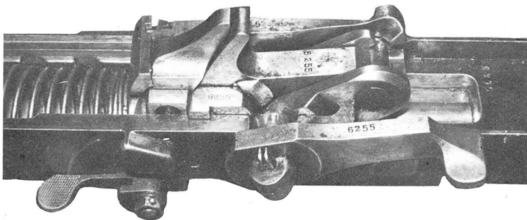
Il meccanismo con il compressore armato e dopo lo sparo.
