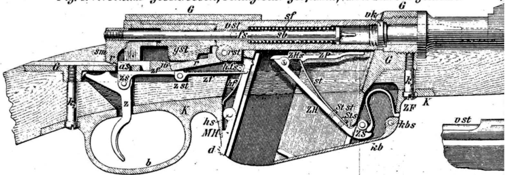
Fig. 3. Verschluß geöffnet, Schlagbolzen gespannt, Magazin eingeführt.
