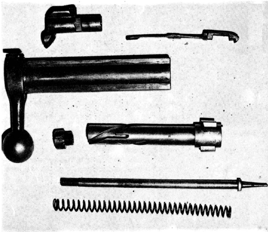
Otturatore smontato.
