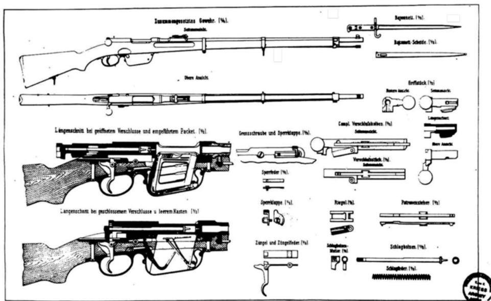
Il Mannlicher modello 1885.
