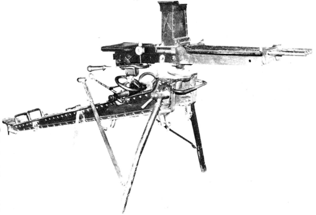
Mitragliera Nordenfelt in calibro 8 mm. austriaco.
