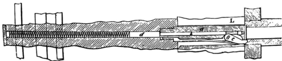
Sezione verticale e orizzontale del sistema.
