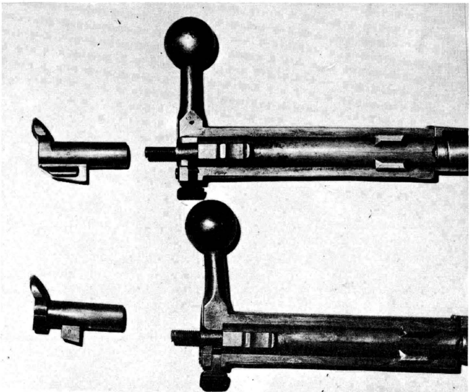
Due tipi di otturatore M 95: in alto, il più vecchio.
