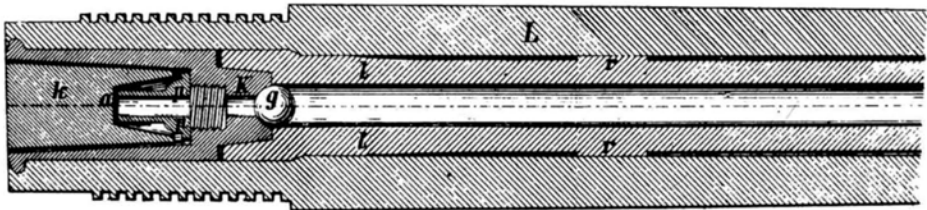
Il «Ladenkanuse» per Zimmergewehr M 1871 e uno spaccato dello Zimmergewehr M 1877.
